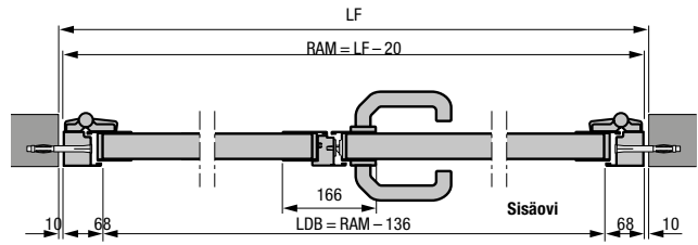
2-lehtinen sivuovi ja alumiininen karmi, profiilityyppi 2 Asennus aukkoon
