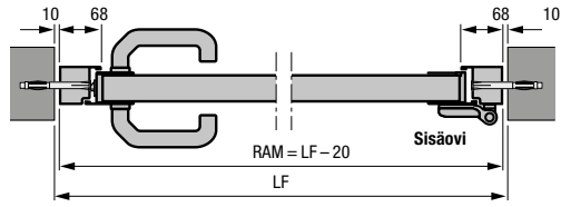
Alumiinisella karmilla varustettu sivuovi, profiilityyppi 2 Asennus aukkoon
